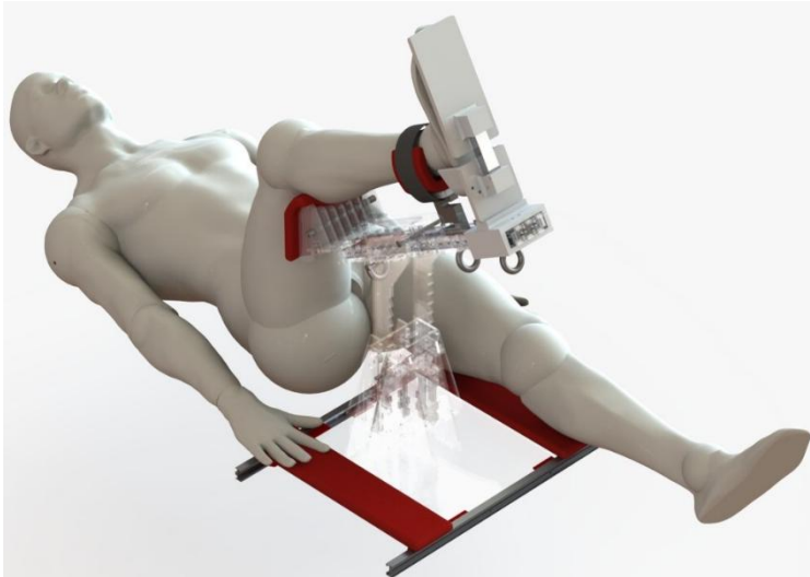
Figura 1. Plataforma de posicionamento de membro para avaliação da força muscular induzida por NMES em paciente crítico.
