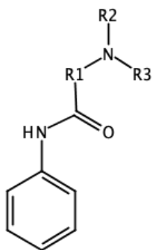
Figura 1- Molécula de aminoamida
