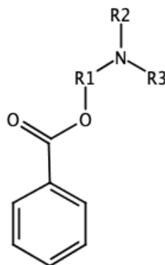
Figura 2- Molécula de aminoéster
