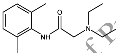
Figura 3 – Molécula de Lidocaína
